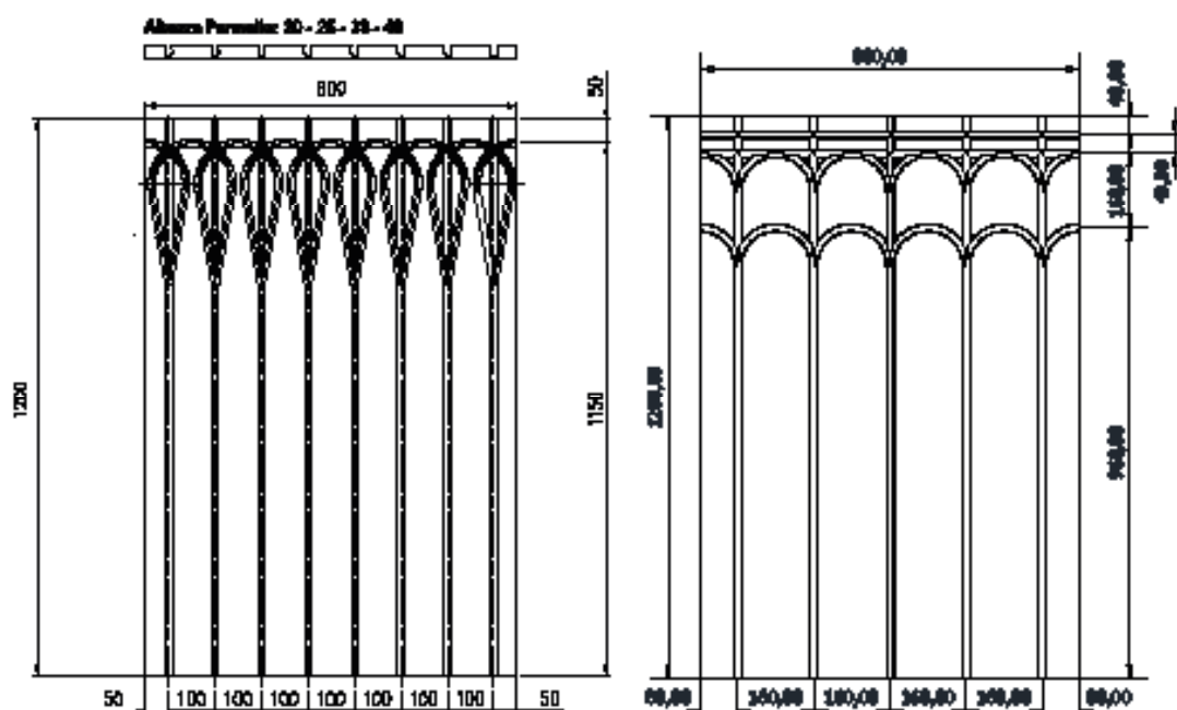
Pannello interasse di posa 100 mm
